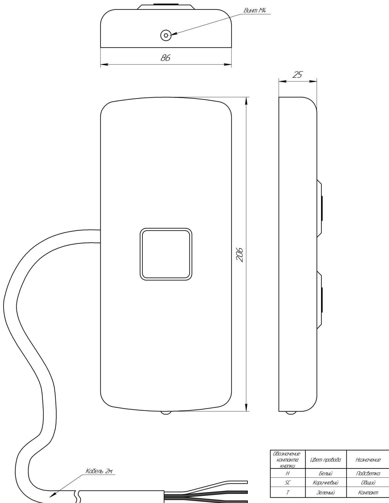
Рис.1 Внешний вид и габаритные размеры Вызывного поста ВП-1000-01
